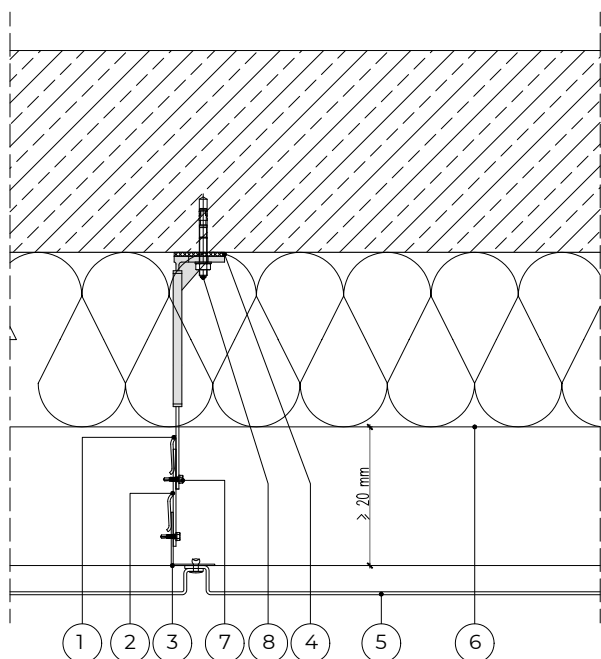
Detal poziomy
