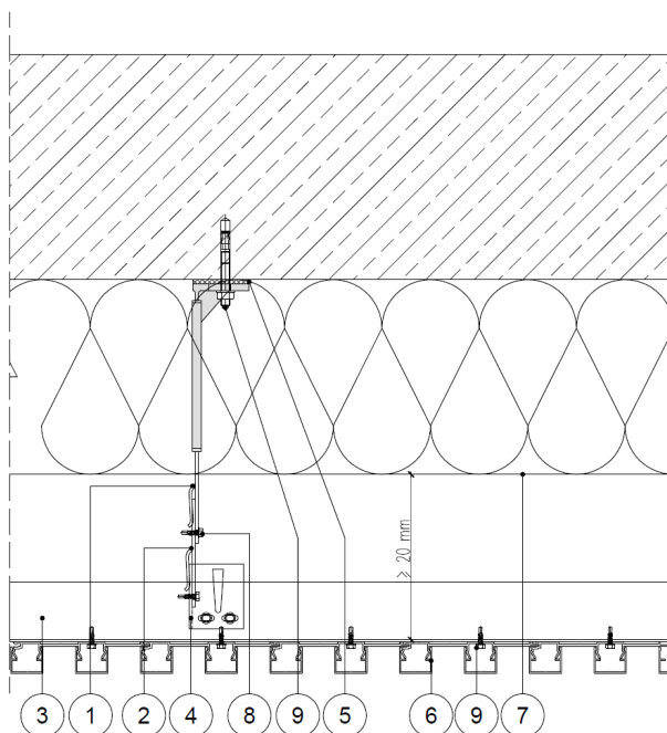
Detal poziomy
