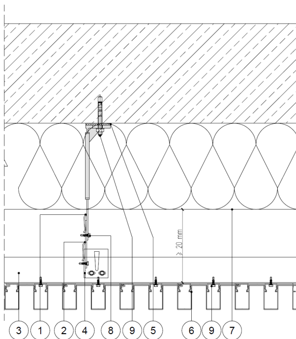
Detal poziomy
