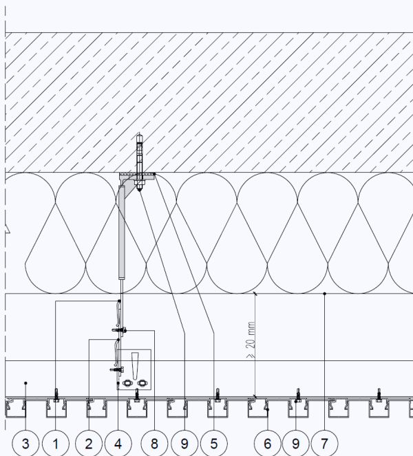
Przykładowy detal poziomy
